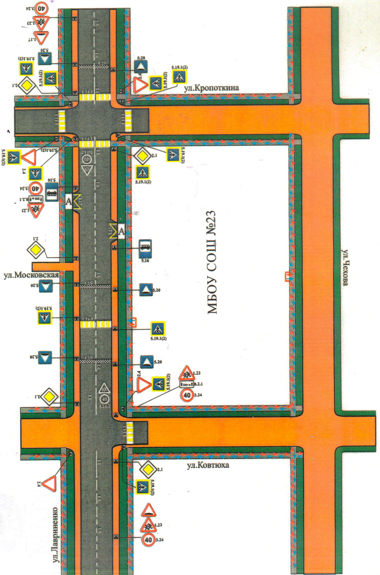
Схема организации дорожного движения в непосредственной близости от образовательного учреждения МБОУ-СОШ №23 с размещением технических средств и маршрута безопасного движения детей
